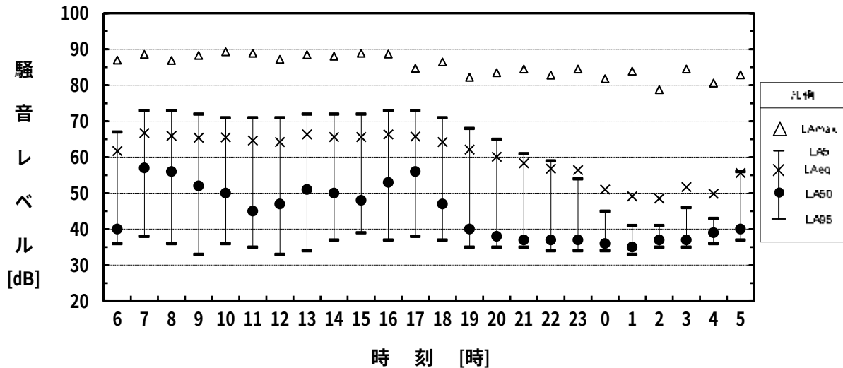
図 2.3-3(1)騒音調査結果 (A. 県道 276 号 (木尾南集落): 平日)
