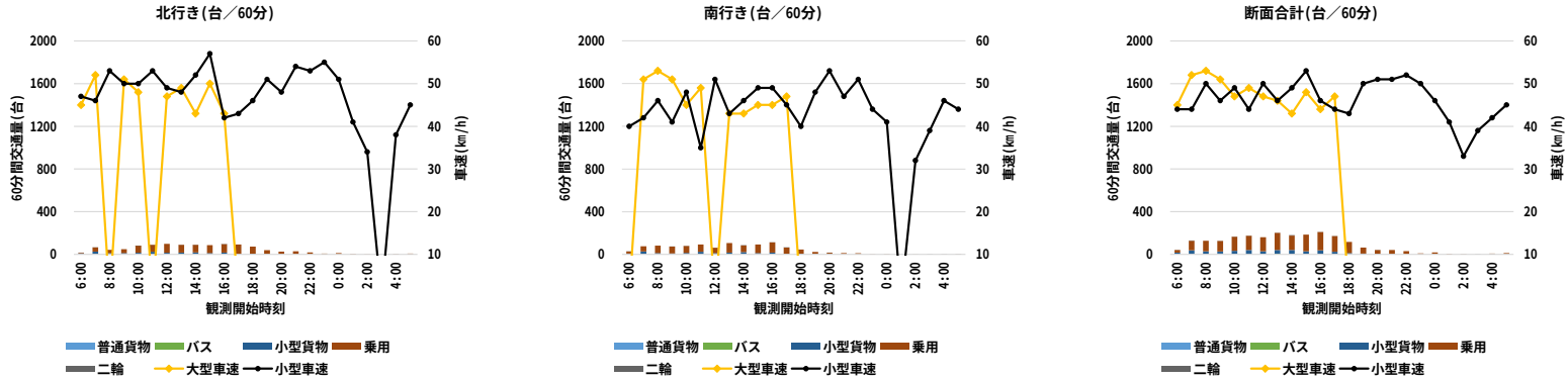
図 2.2-1(2)交通量測定結果 (A. 県道 276 号 (木尾南集落)：休日)
