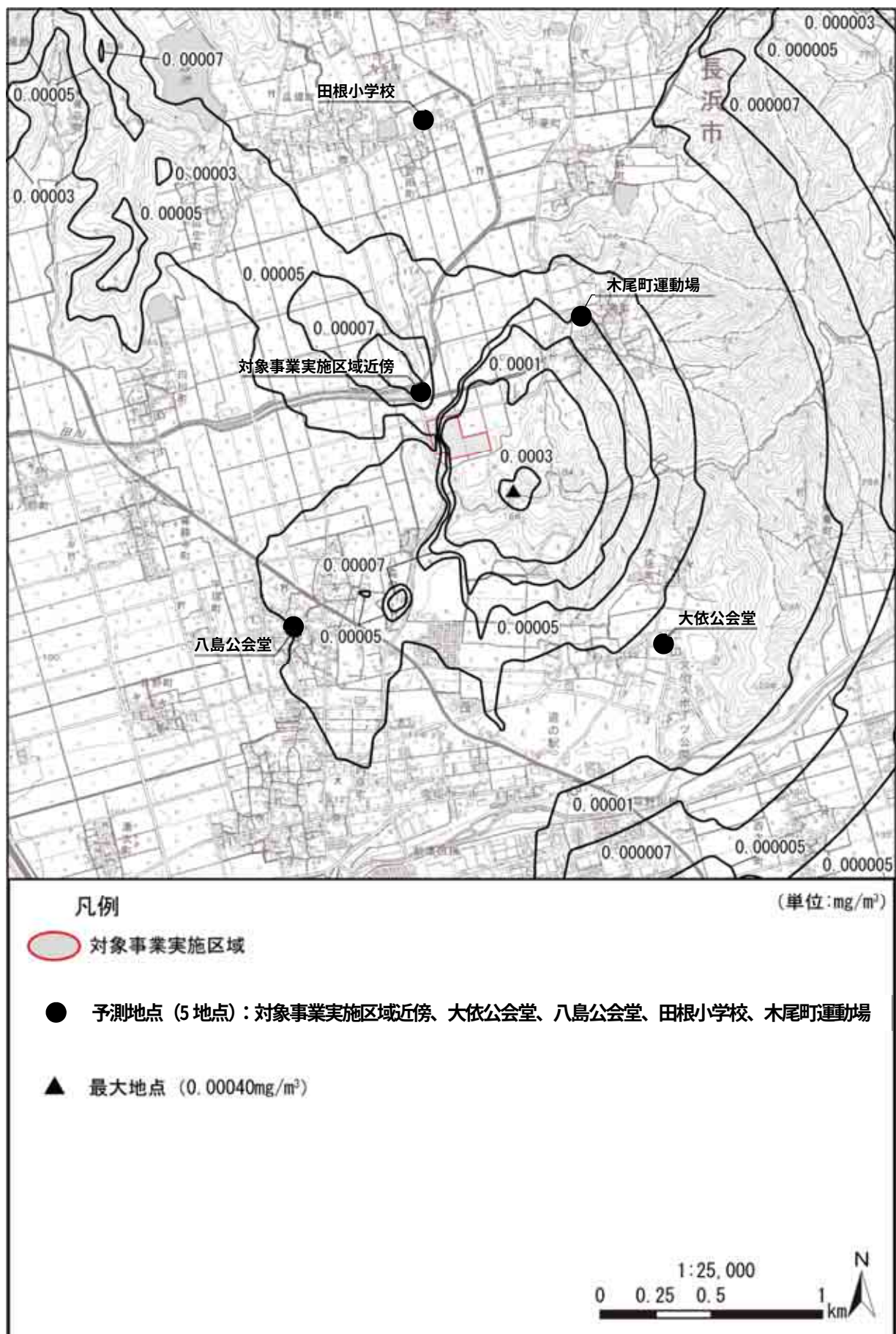
図 3.1-4(3) 複合時の長期平均濃度予測結果[浮遊粒子状物質 (年平均値)] (寄与分:補正あり)
