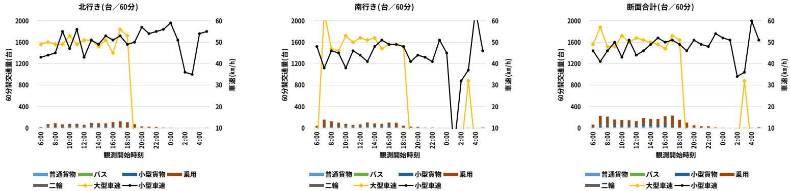
図 2.2-1(1)交通量測定結果 (A.県道 276 号 (木尾南集落)：平日)
