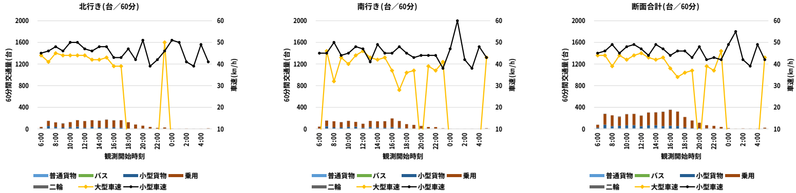
図 2.2-3(2)交通量測定結果（C.県道 276 号（浅井体育館）：休日）
