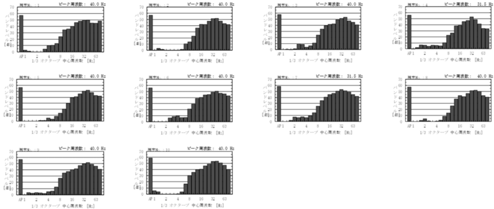
図 2.5-8 地盤卓越振動数調査結果（C.県道 276 号（浅井体育館）：平日）
