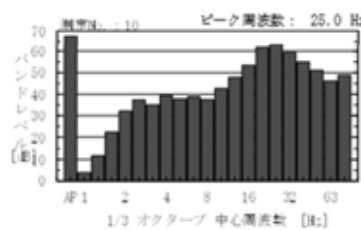
図 2.5-6 地盤卓越振動数調査結果 (A.県道 276 号 (木尾南集落): 平日)
