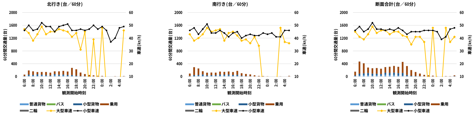
図 2.2-3(1)交通量測定結果（C.県道 276 号（浅井体育館）：平日）
