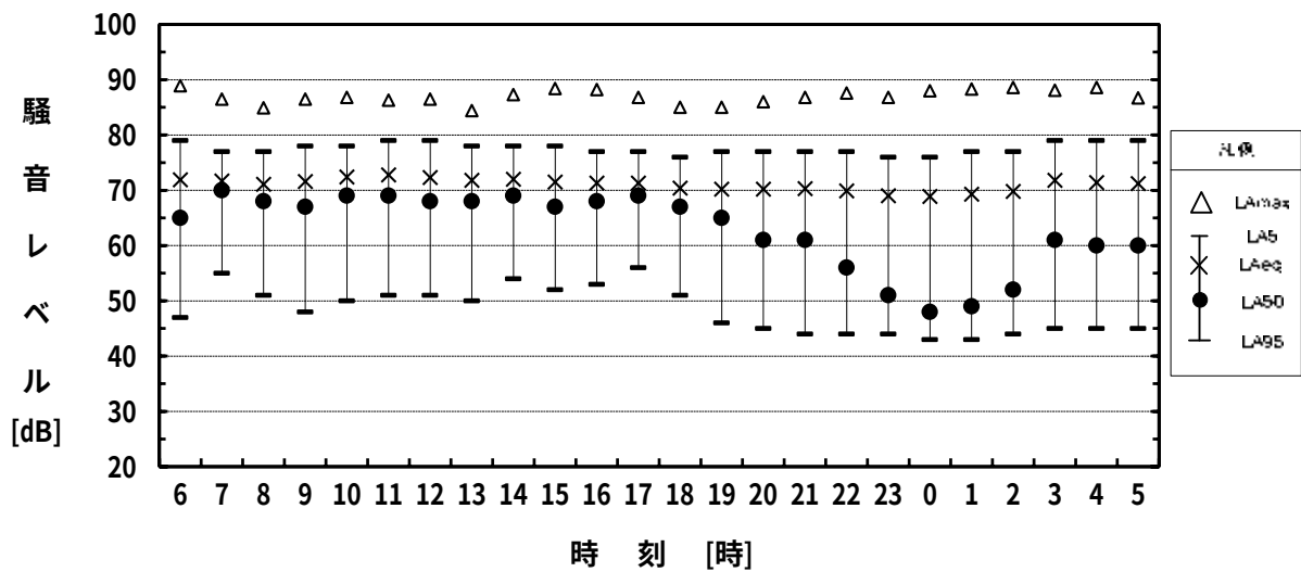
図 2.3-4(1)騒音調査結果 (B.国道 365 号 (浅井福祉センター) : 平日)
