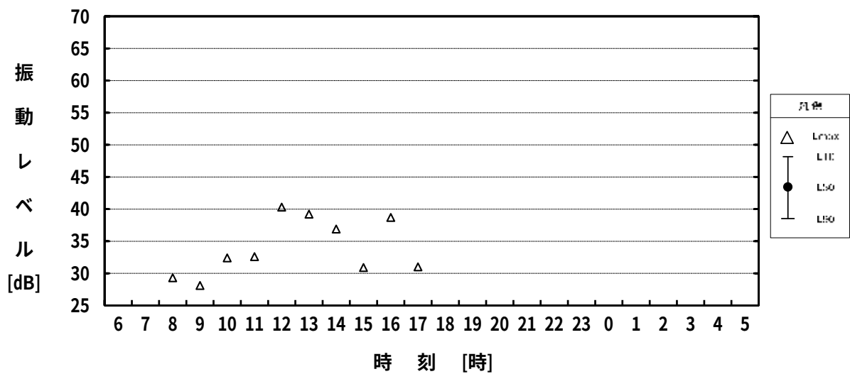
図 2.5-2(1)振動調査結果 (1.対象事業実施区域近傍：平日)
