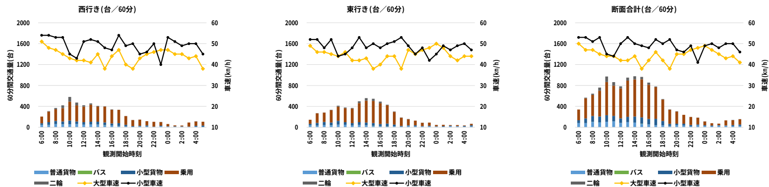
図 2.2-2(2) 交通量測定結果 (B. 国道 365 号 (浅井福祉センター) : 休日)
