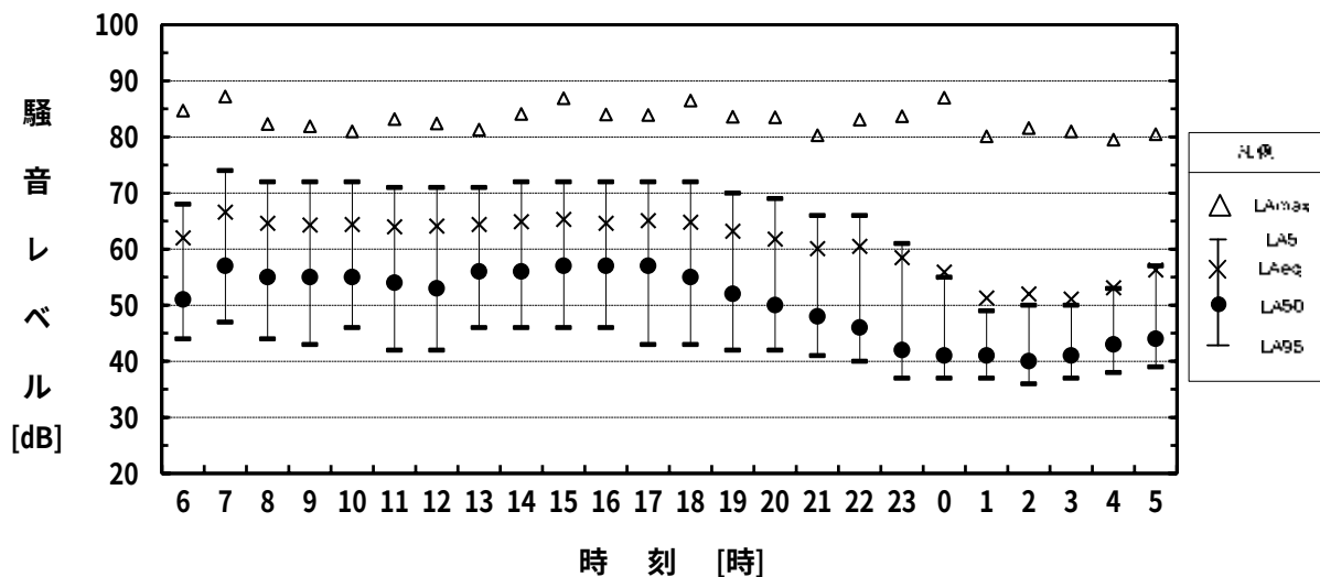
図 2.3-5(2)騒音調査結果 (C. 県道 276 号 (浅井体育館): 休日)
