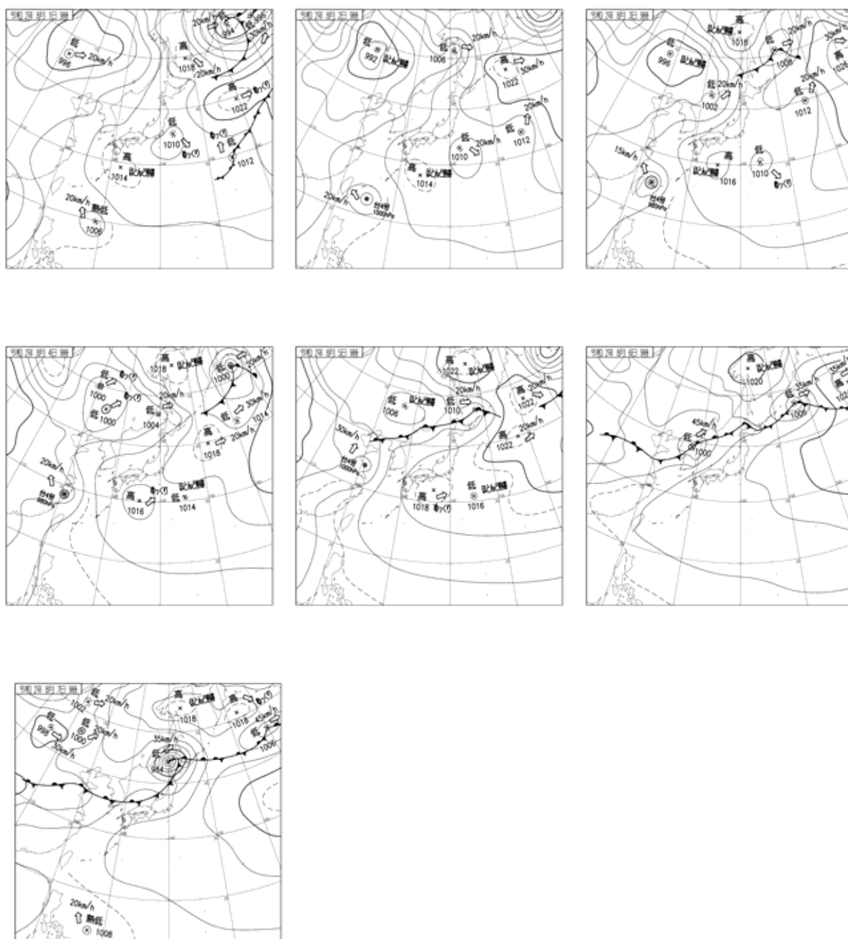
図 2.1.2-2(3) 観測期間中の天気図（夏季）
