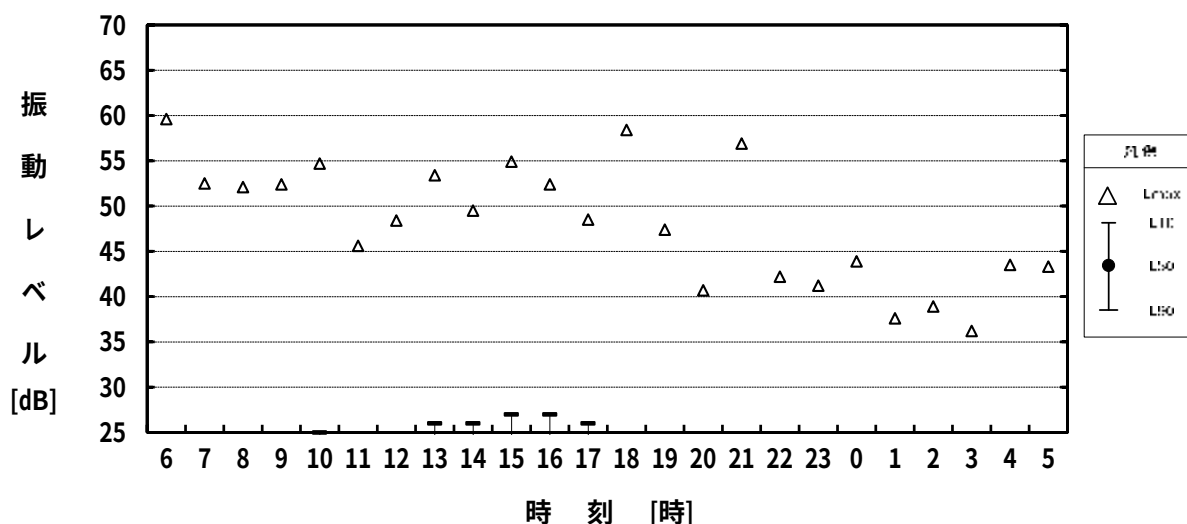
図 2.5-3(2)振動調査結果 (A. 県道 276 号 (木尾南集落)：休日)
