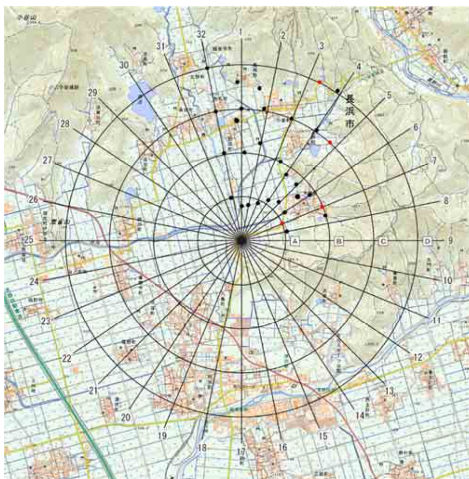
図 2.1.3-3(5) 各アークの最大濃度地点（夏季）
