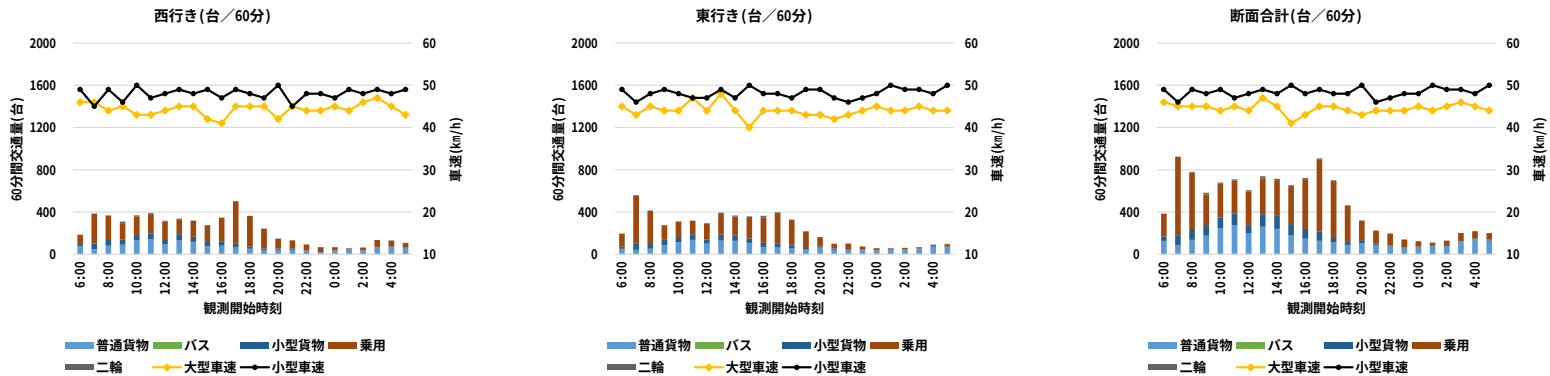
図 2.2-2(1)交通量測定結果 (B.国道 365 号 (浅井福祉センター)：平日)
