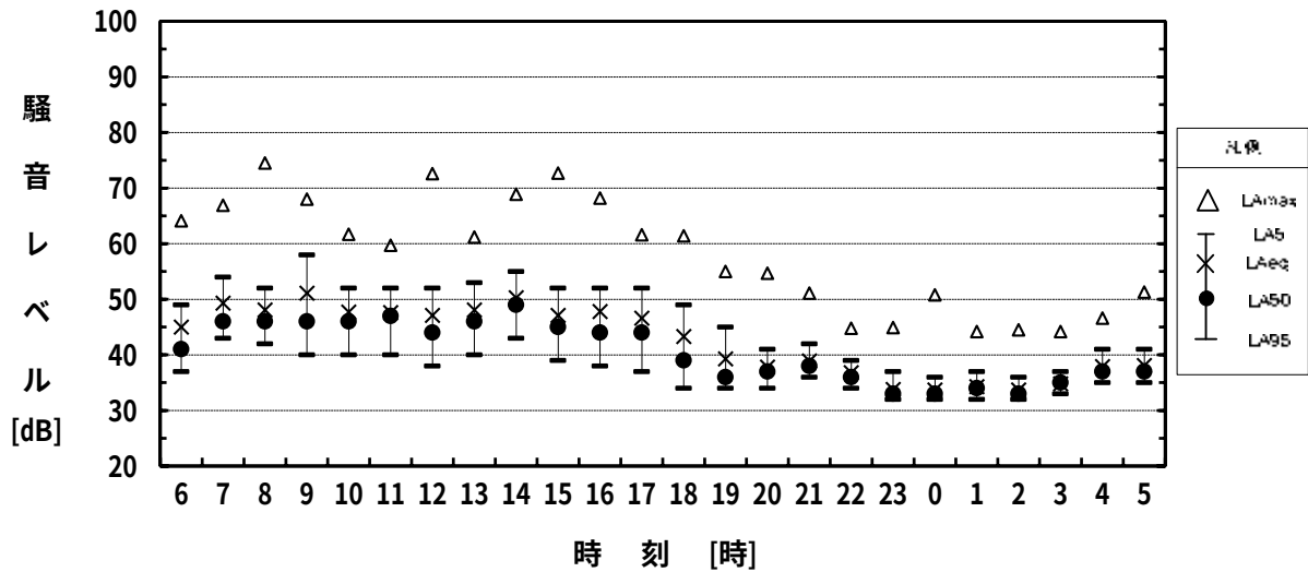
図 2.3-1(2)騒音調査結果（対象事業実施区域敷地境界：休日）
