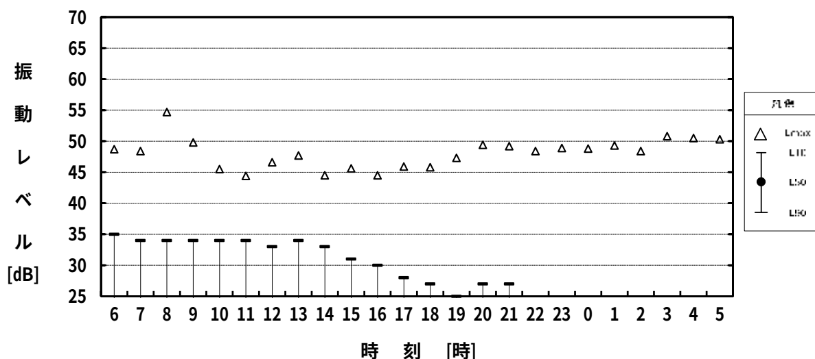
図 2.5-4(2) 振動調査結果 (B. 国道 365 号 (浅井福祉センター) : 休日)
