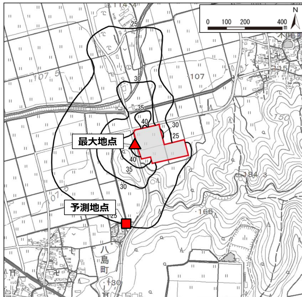
供用後の騒音予測地点と最大地点位置(昼間)
